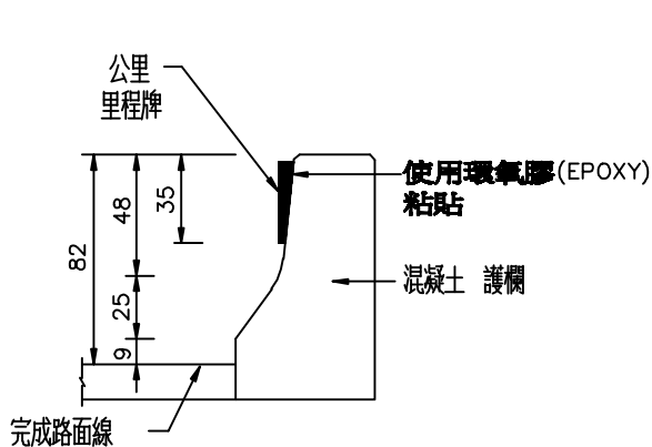
黏貼式公里里程牌 (C型)
