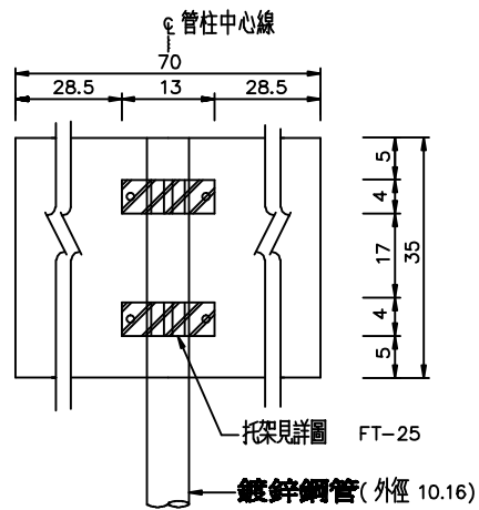
牌面安裝詳圖 (公里)
